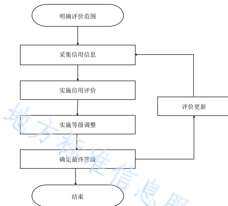
图 1 评价流程
